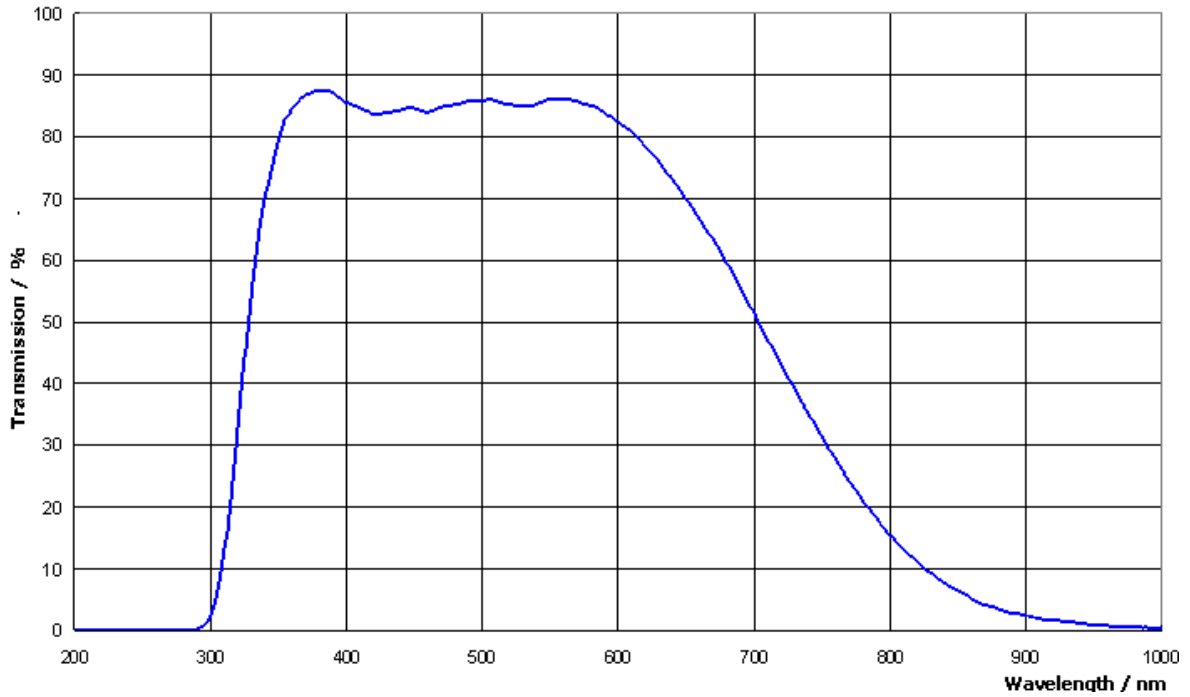
KG 1, IR - range, th 3 mm
